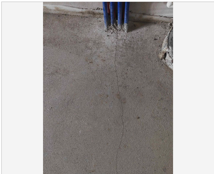
Г.тверь жк Онегин · Кв. Г.тверь жк Онегин — 14.10.2026 · Трещины на поверхности бетона (до 0,2 мм)
