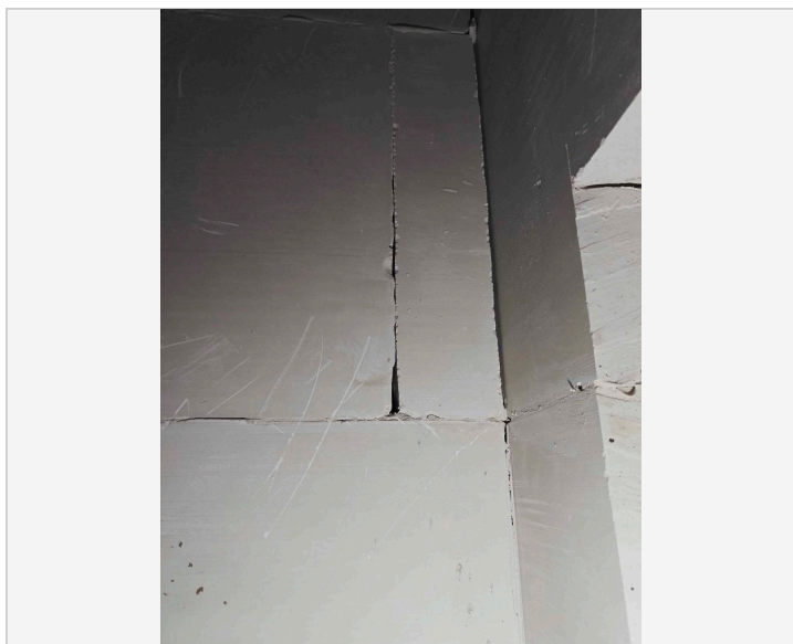
Г.тверь жк Онегин · Кв. Г.тверь жк Онегин — 14.10.2026 · Глубина незаполненных швов кладки (до 15 мм)
